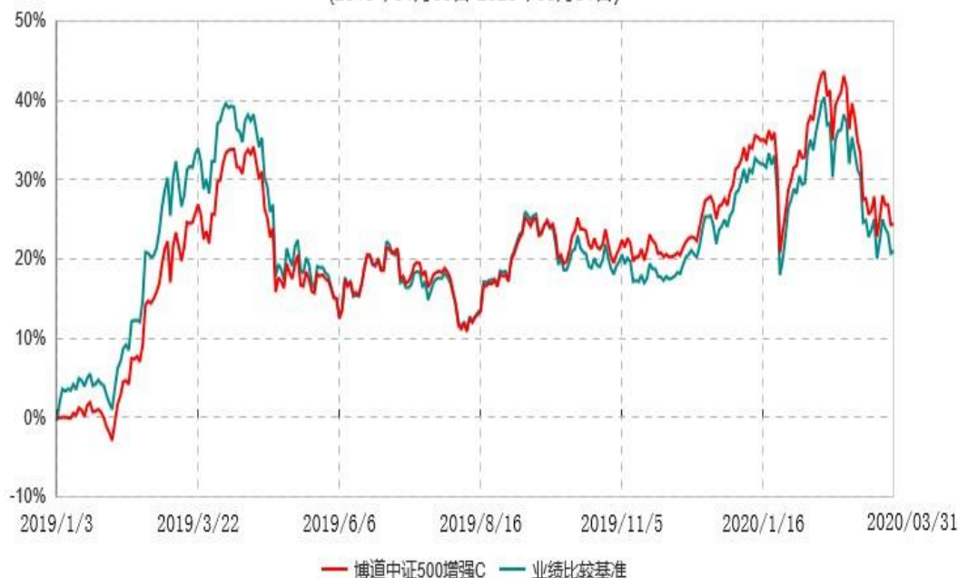
博道中证500增强C累计净值增长率与业绩比较基准收益率历史走势对比图
